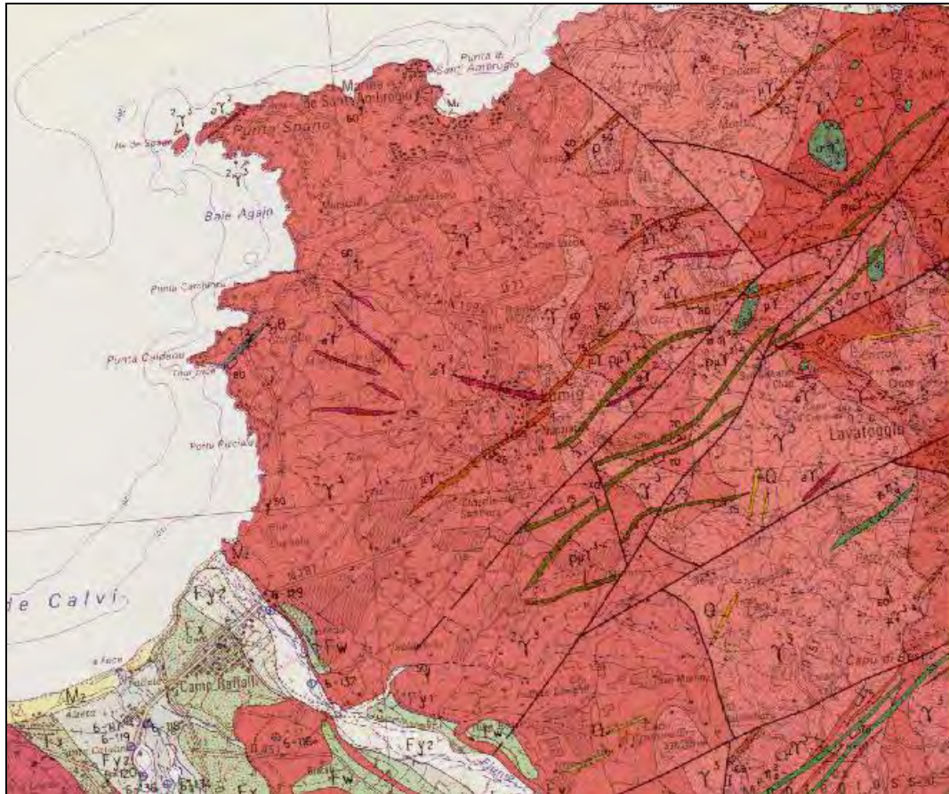
Extrait de la carte géologique de Calvi au 1/50 000 (BRGM)
